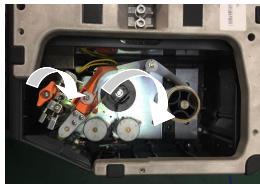
(4) 将纸卷前段绕过过滤板卷入收纸轴，合上打印头（如上图）
