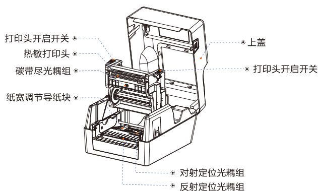
□ 内视图
