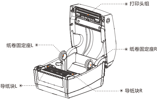
内视图
