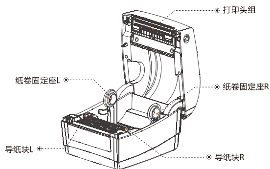
❑ 内视图
