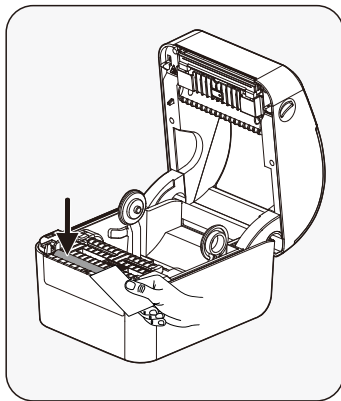
清洁打印机胶辊示意图
