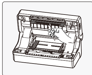
清洁打印头示意图
