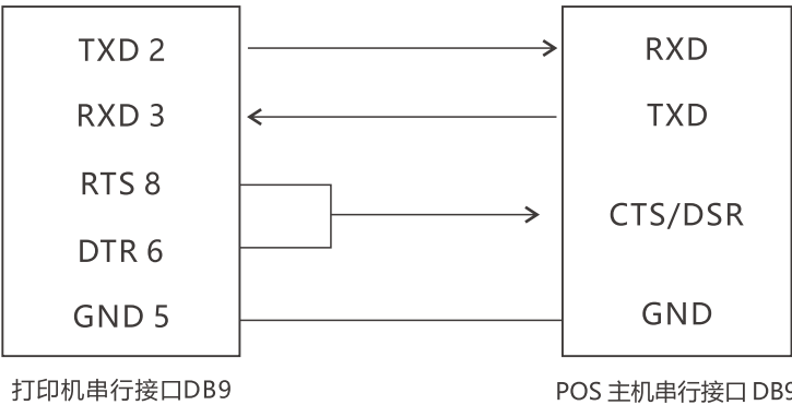
打印机串行接口与 POS 主机串行接口连接示意图：
