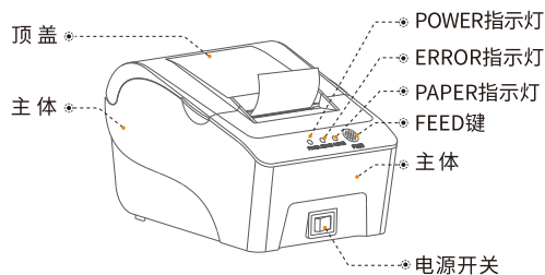
前视图
