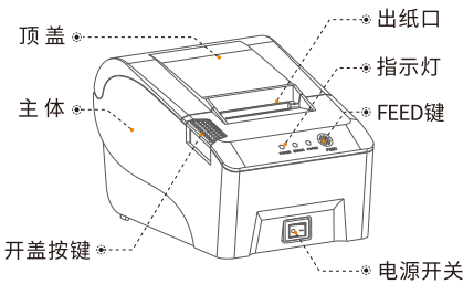
前视图
