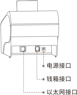
后视图
