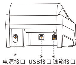
后视图
