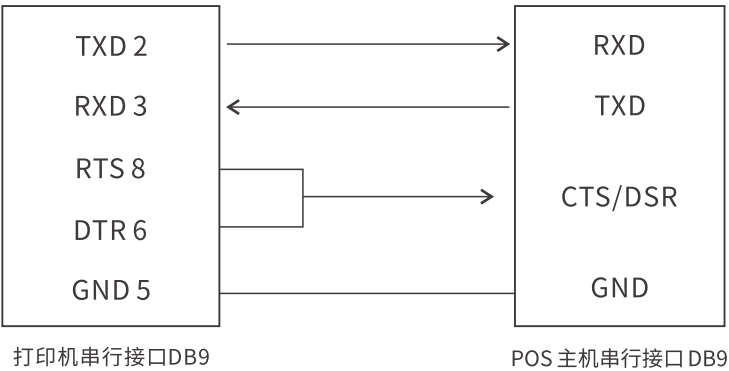
打印机串行接口与 POS 主机串行接口连接示意图:
