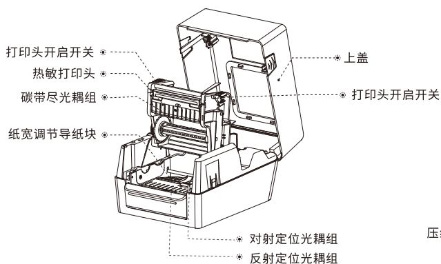
内视图
