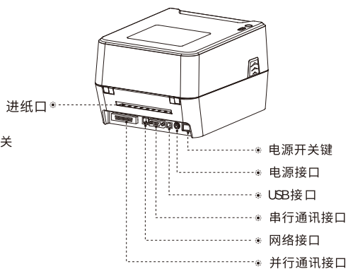
后视图
